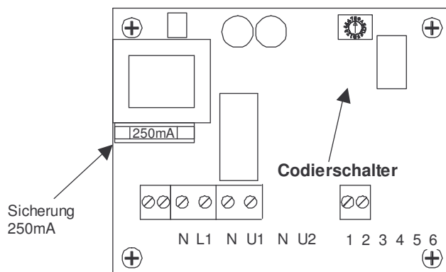
Bild 2. Platine
